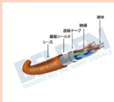
IEF-FIX01 固定部 単線タイプ
