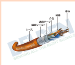
IEF-FLX01 固定部 撚線タイプ
